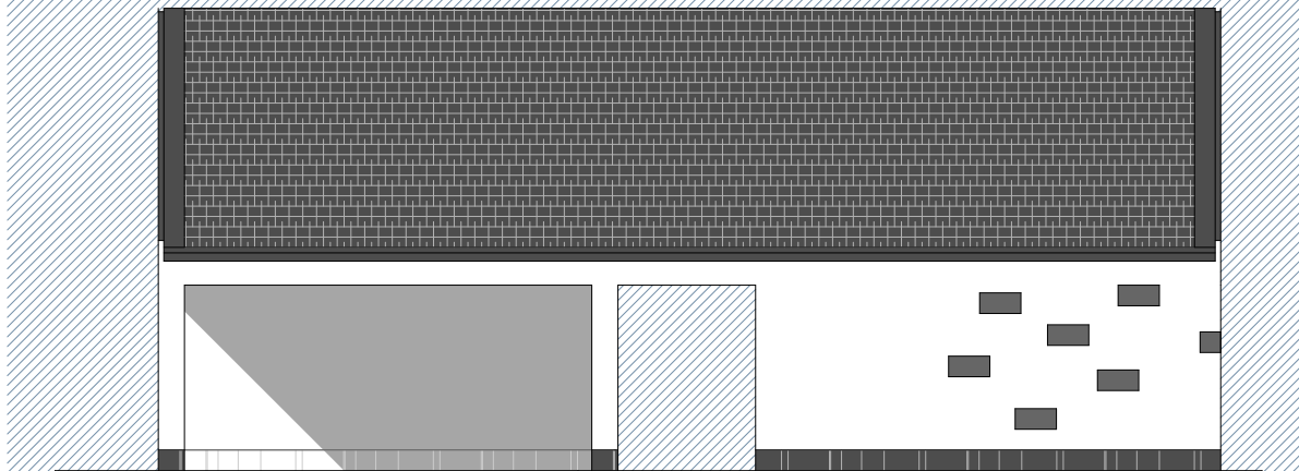
DÉLKELETI HOMLOKZAT
