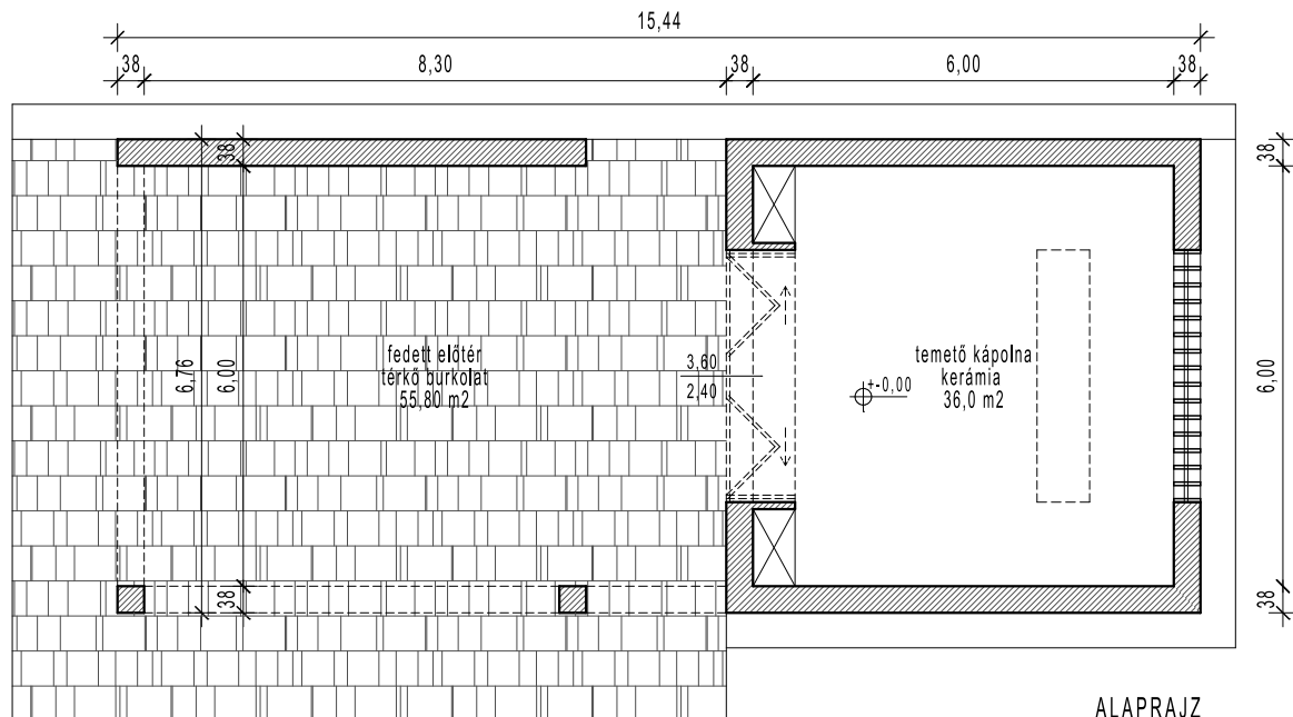
ALAPRAJZ
