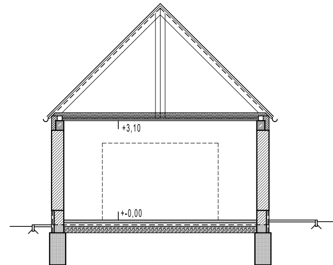
KERESZTMETSZET
