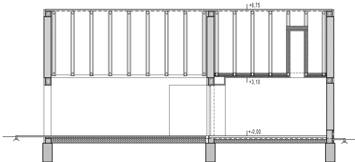
HOSSZMETSZET
